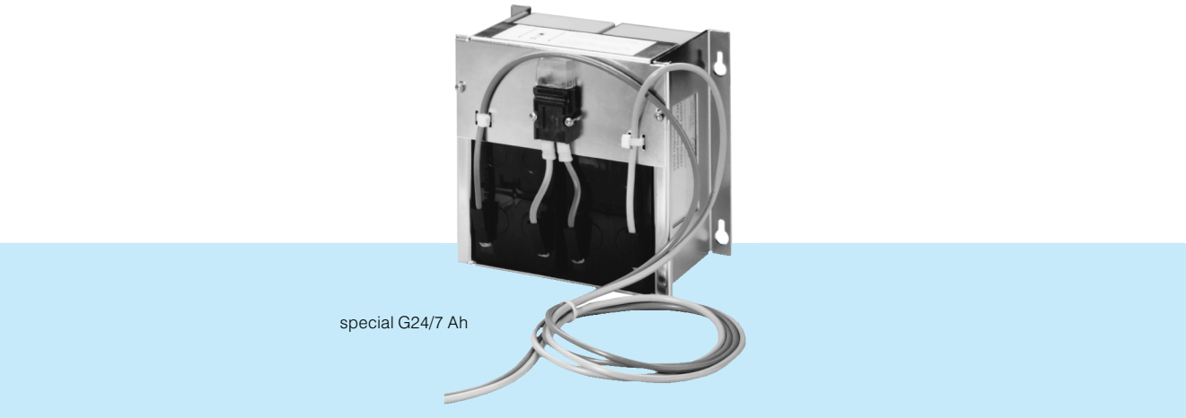
Bild 3/13 Batteriemodul 7 Ah für Unterbrechungsfreie Stromversorgung
